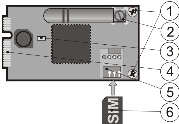
1. ábra: A JA-194Y kommunikátor - Főbb elemek: 1 – rögzítő csavarok; 2 – a GSM antenna SMA csatlakozója; 3 – a zöld visszajelző LED mutatja a működő GSM kapcsolatot meglétét; 4 – rendszer csatlakozó; 5 - SIM kártya tartó; 6 – SIM kártya
